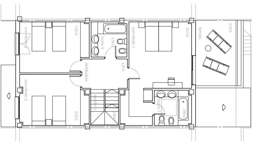
Planta Primera
